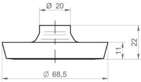
D04-66 DIN 11851 (mlékárenské šroubení) DN50 (BCID: D04)
