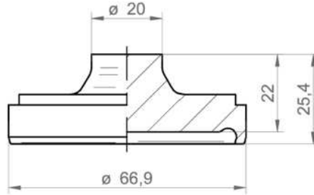
H04-68 DIN 11864-1-A (aseptické šroubovací) DN50 (BCID: H04)
