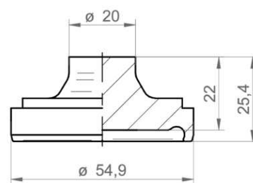
H03-59 DIN 11864-1-A (aseptické šroubovací) DN40 (BCID: H03)
